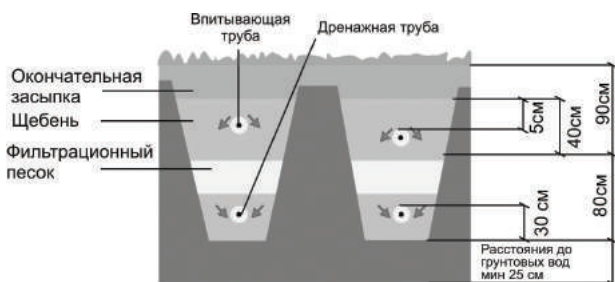
Рис. 6 Поперечное сечение фильтрующей площадки
