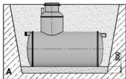
Рис. 3 Схема монтажа
