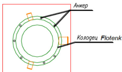
Нижняя ж/б плита
