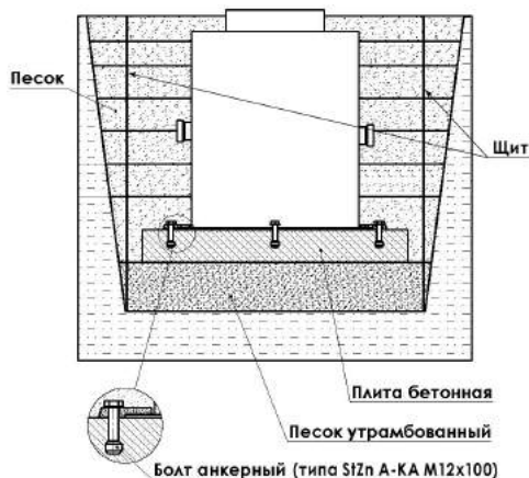
Рис. 3 Расположение бетонной плиты
