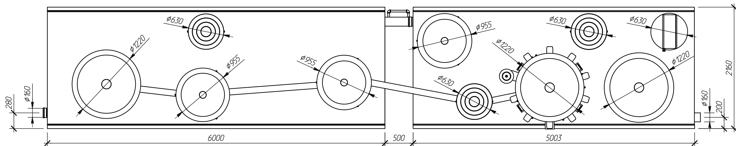
Вид сверху
